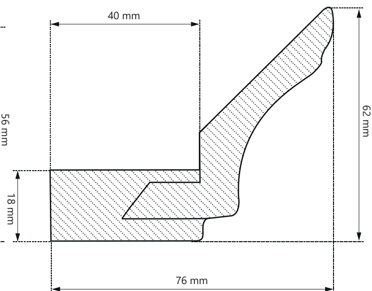
Listwa B2 - listwa z wklejoną podstawą
